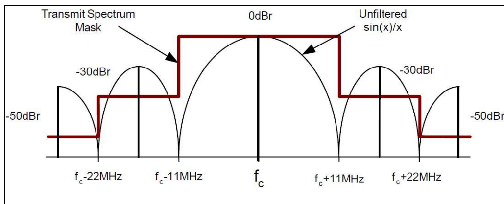
IEEE 802.11b Spectral Mask
