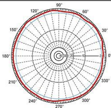
H-Plane Pattern
